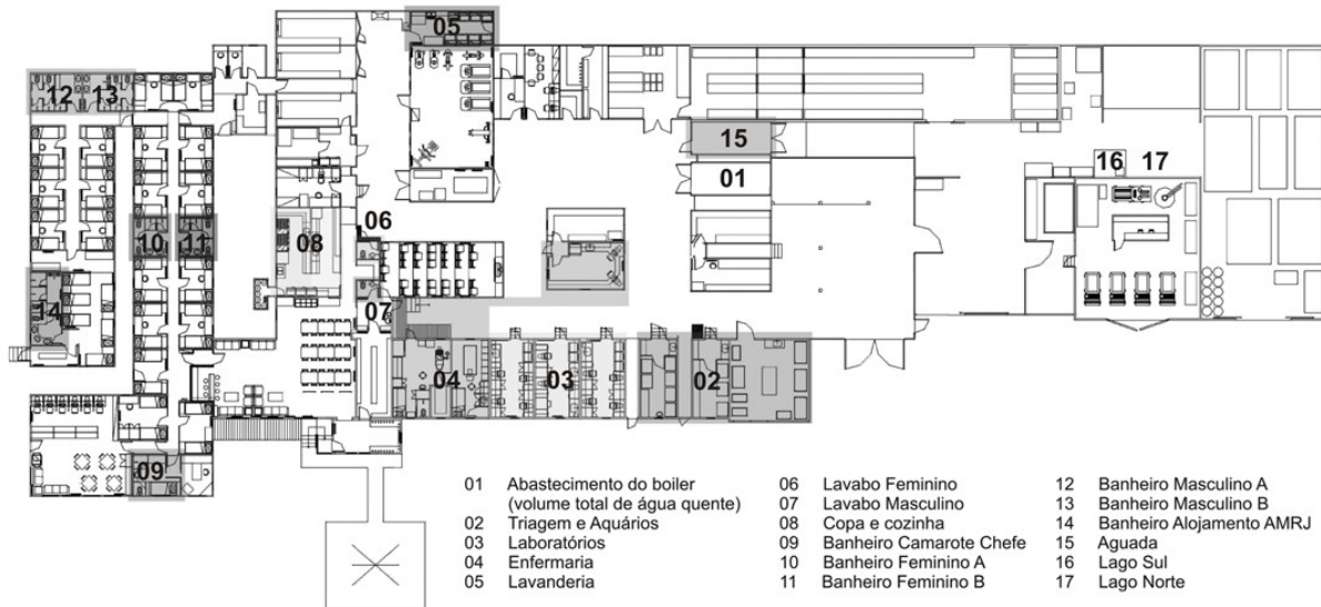
Figura 3. Planta de setorização do consumo de água da EACF
