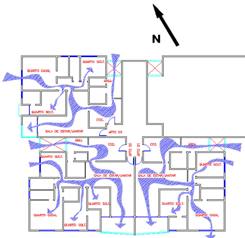
Figura 59: representação do percurso do vento elaborado a partir das respostas aos questionários aplicados aos usuários e da avaliação técnica no EDIFÍCIO 02.
