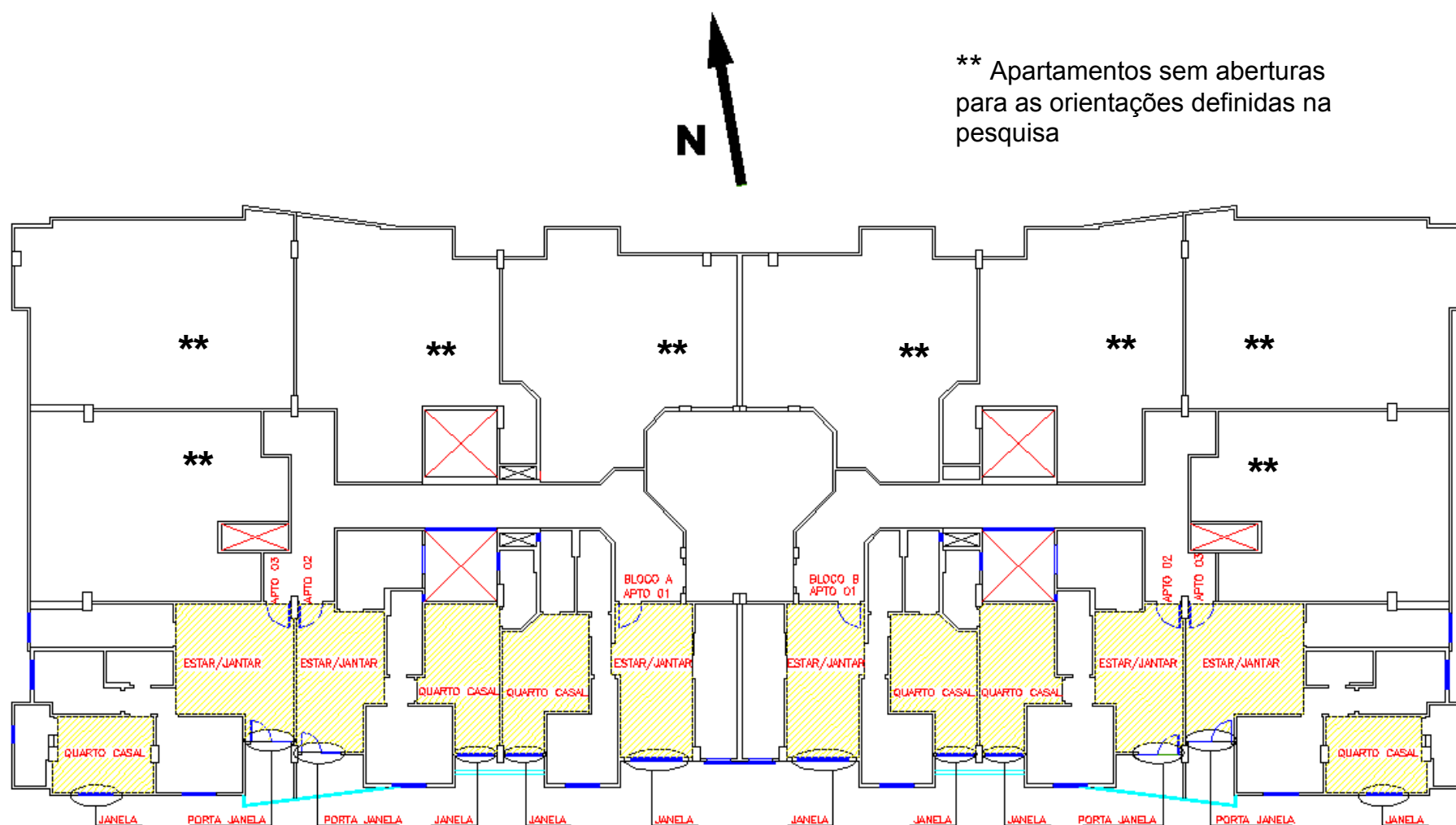
Figura 52: planta baixa com a localização dos ambientes e das janelas no EDIFÍCIO 01. Fonte: Construtora Morar, arquiteto Kennedy P C R Vianna, 2003.
