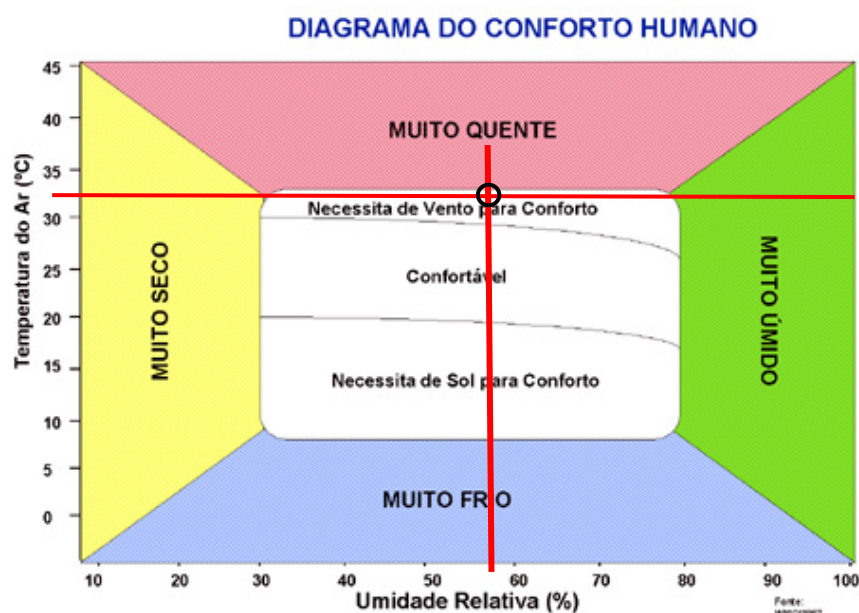
Gráfico 2: diagrama para a definição do conforto humano em Vitória com relação à temperatura e a umidade relativa do ar.
