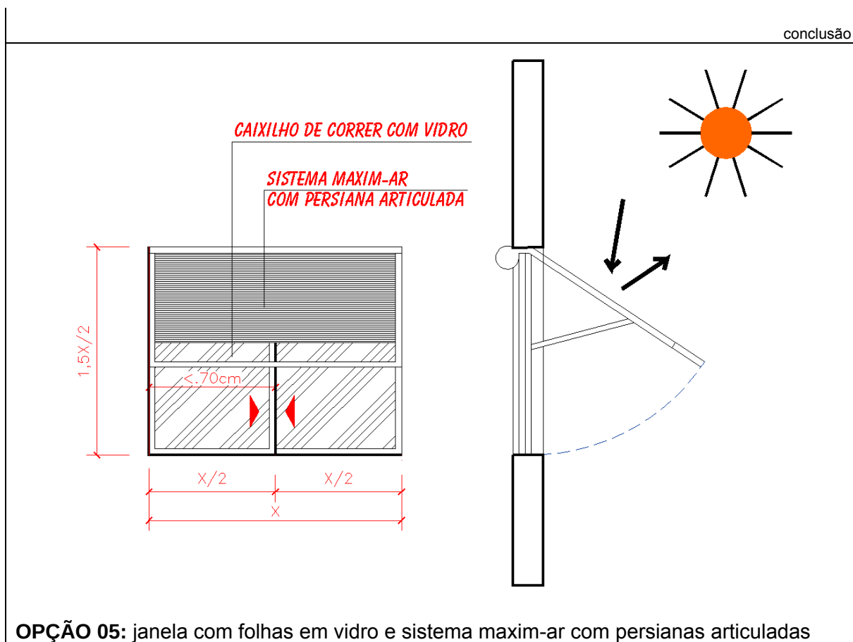
Quadro 19: 1ª proposta de tipologia de janela com as variações dos elementos.
